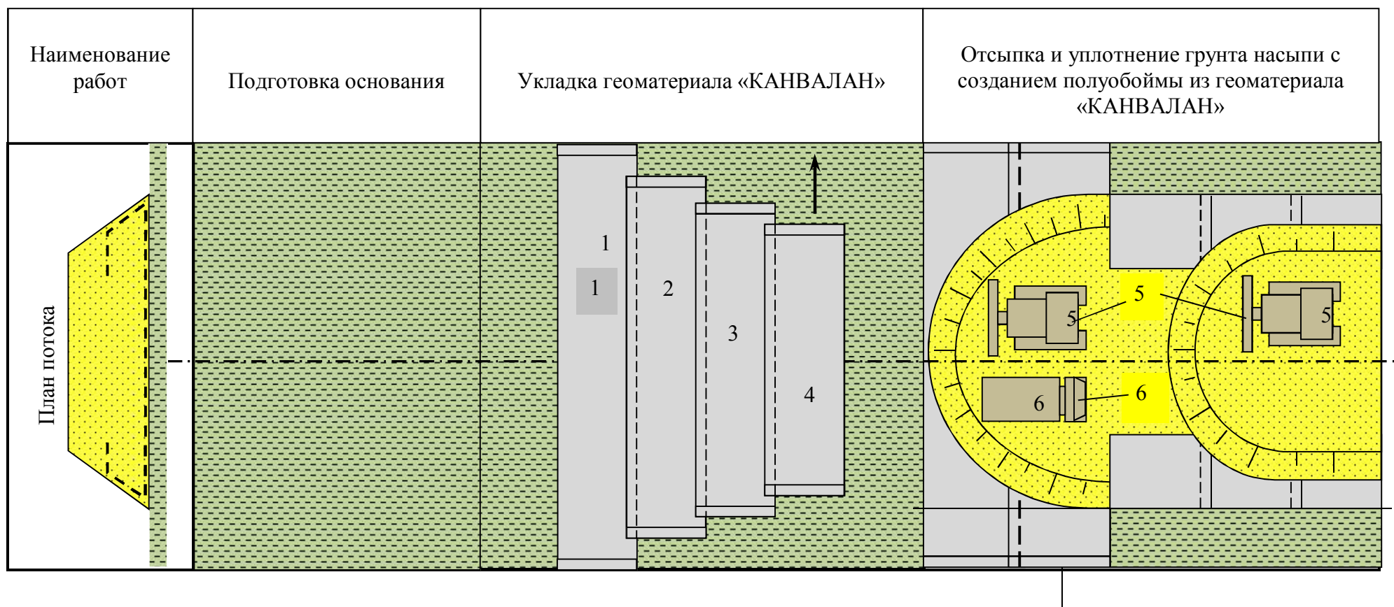
Рис. 3. Технологическая схема по устройству разделяющих и армирующих прослоек из геоматериала «КАНВАЛАН» на слабом основании: 1-4 – ГМ; 5 – бульдозер; 6 – автомобиль-самосвал.
